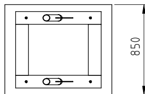
Skizze 2: Fundamentplan
