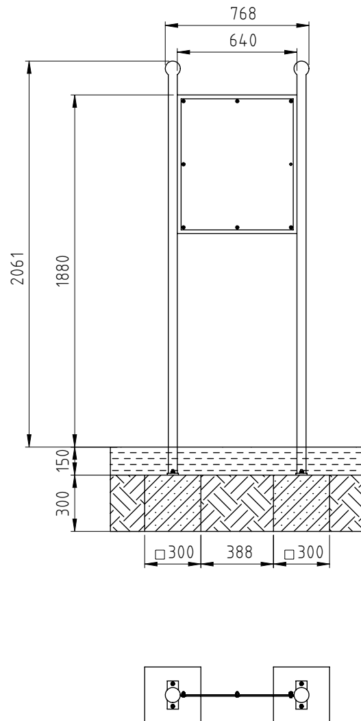
Skizze 4: Fundamentplan Instruktionsstafel
